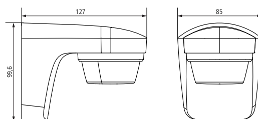
Plan d'encombrement
